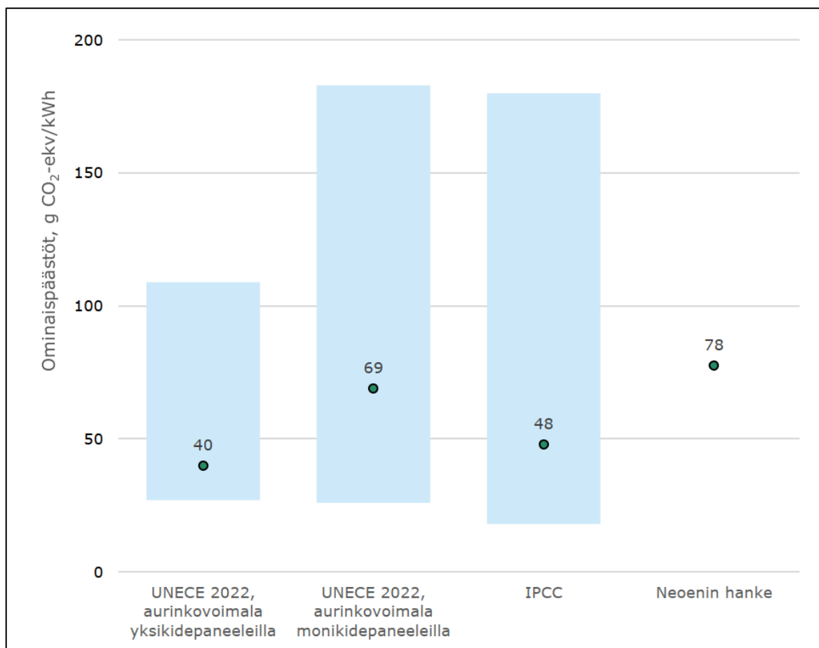
Kuva 10.7 Kansainvälisesti toteutettujen aurinkovoimahankkeiden ominaispäästöjen vaihteluvä- lejä sekä Neoenin Kerkkolan hankkeen ominaispäästö. Pisteet kuvaavat keskiarvoja.
