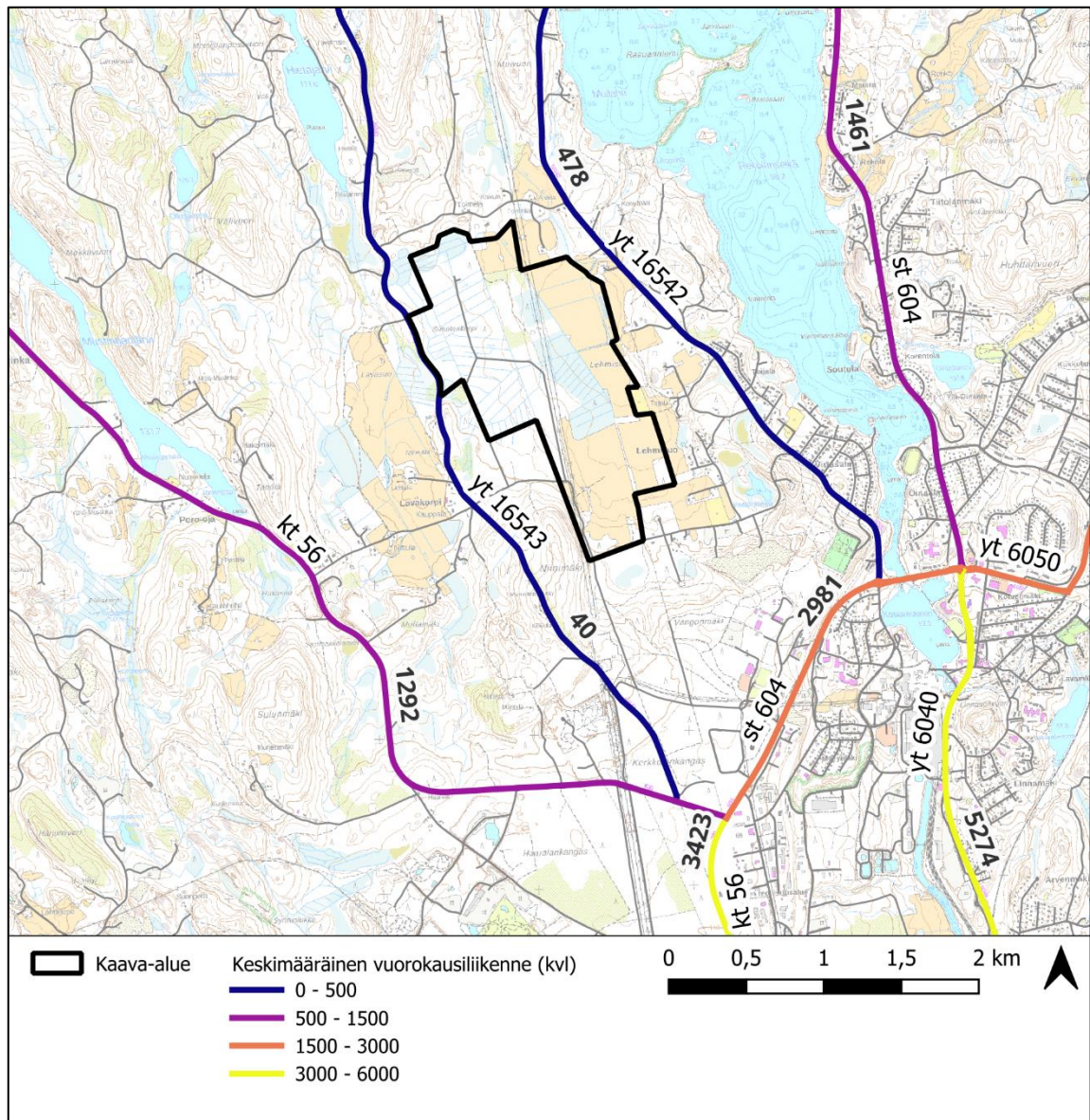
Kuva 4.7 Kaava-alueen ja sen lähistön tärkeimmät tiet sekä niiden keskivuorokausiliikenne. (Digiroad, 2023)
