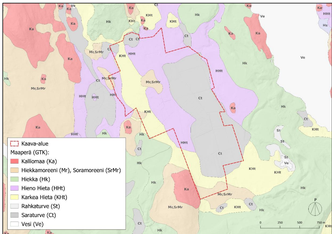
Kuva 8. Hankealueen maaperä (maaperäkartta: GTK).
