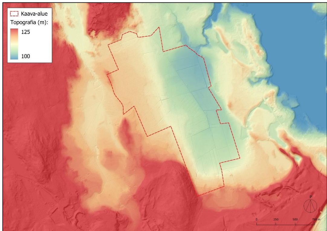
Kuva 7. Hankealueen topografia (korkeusmalli: MML).
