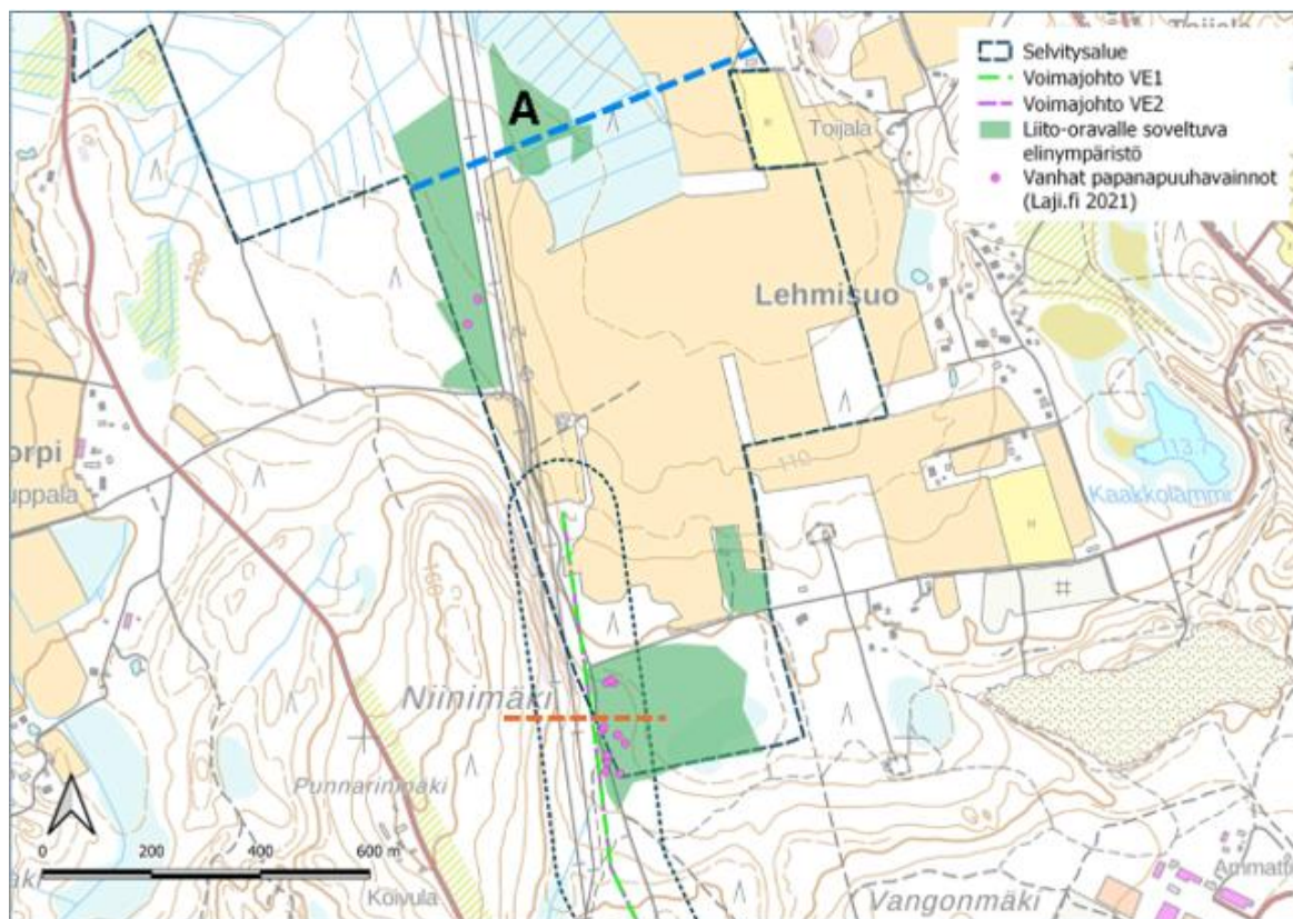
Kuva 10.8 Mahdollinen ekologisen käytävän sijainti, sininen katkoviiva. Oranssi katkoviiva yhteisvaikutuksia lieventävä ekologinen käytävävaihtoehto (ks. Kappale 10.17). Liito-oravaselvityksen selvitysalue on kaava-alueetta laajempi.
