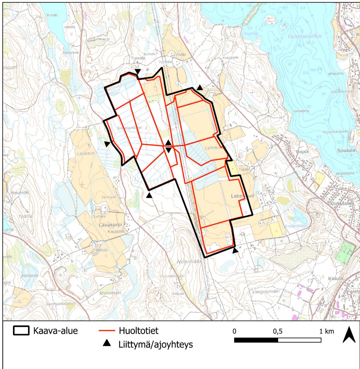
Kuva 7.1 Alustavat ajoyhteudet ja liittymät paneelialueille. Alueen sisäiset huoltotiet (kuvassa punaisella) eivät ole yleisessä käytössä. Huoltoteiden sijaintiin vaikuttaa voimalaan aikanaan valittu paneelityyppi. Voimajohtoalueen nykyisiltä teiltä on mahdollista toteuttaa ajoyhteys aidatulle paneelialueelle kaava-alueen keskiosaan.
