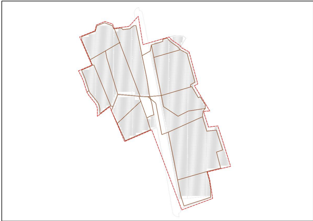
Kuva 2. Hankealueen alustavat paneelialueet 2 , huoltotiet 3 ja kaava-alueen rajausta punaisella. Paneelialueita on tarkennettu vesienhallintasuunnitelmassa (Liite 6-1) ja alueet tarkentuvat edelleen jatkosuunnittelussa.
