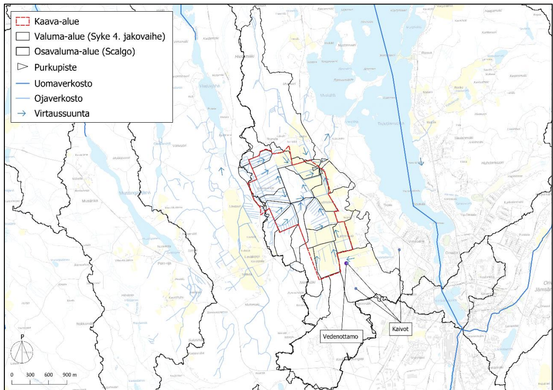
Kuva 5. Hankealueen nykyiset valuma-alueet ja virtausreitit sekä läheisen pohjavesialueen pumppaamo ja kaivot (taustakartta: MML).
