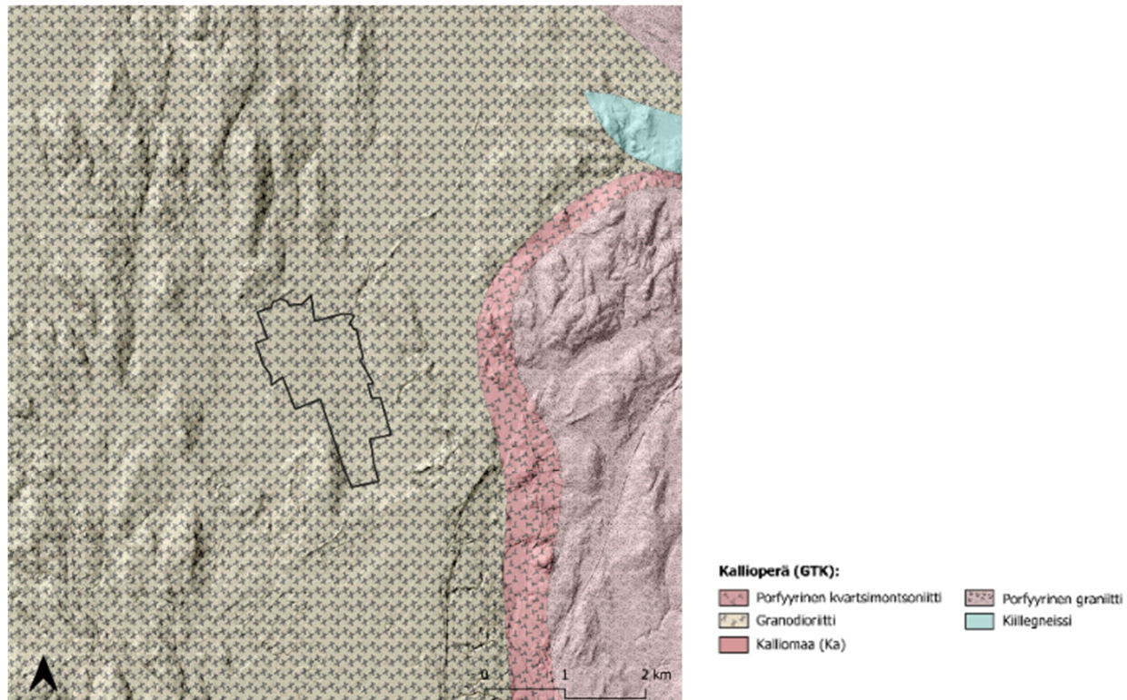
Kuva 10: Kaava-alue on osoitettu mustalla aluerajauksella. Kallioperä on koko kaava-alueella ja sen ympäristössä granodioriittia, joka on tyypillinen keskusomalainen syväkivilaji. Kaava-alueen rajausta kaavaluonnosvaiheen mukaan.
