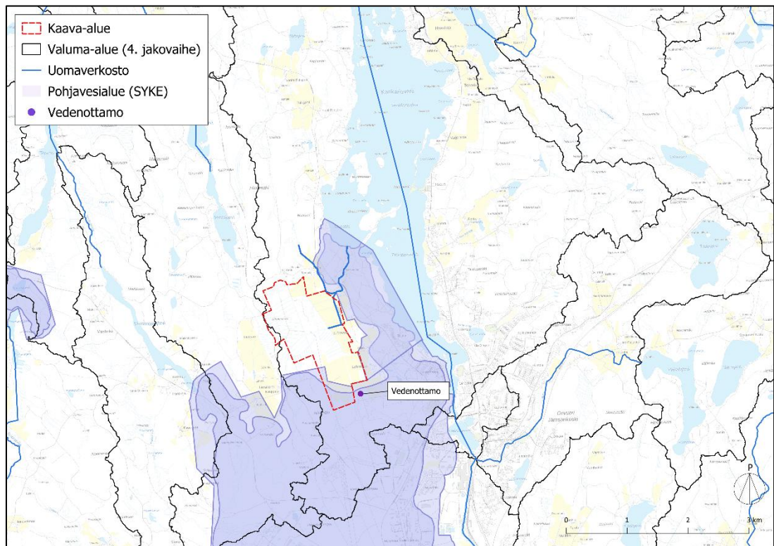
Kuva 3. Hankealueen sijainti valuma-alueilla ja pohjavesialueiden läheisyydessä (taustakartta: MML).
