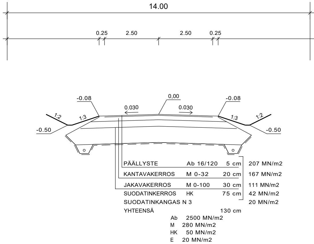
TYYPPIPOIKKILEIKKAUS 1:100
