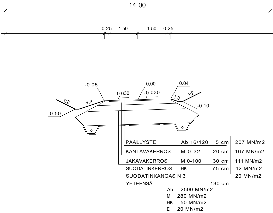
TYYPPIPOIKKILEIKKAUS 1:100
