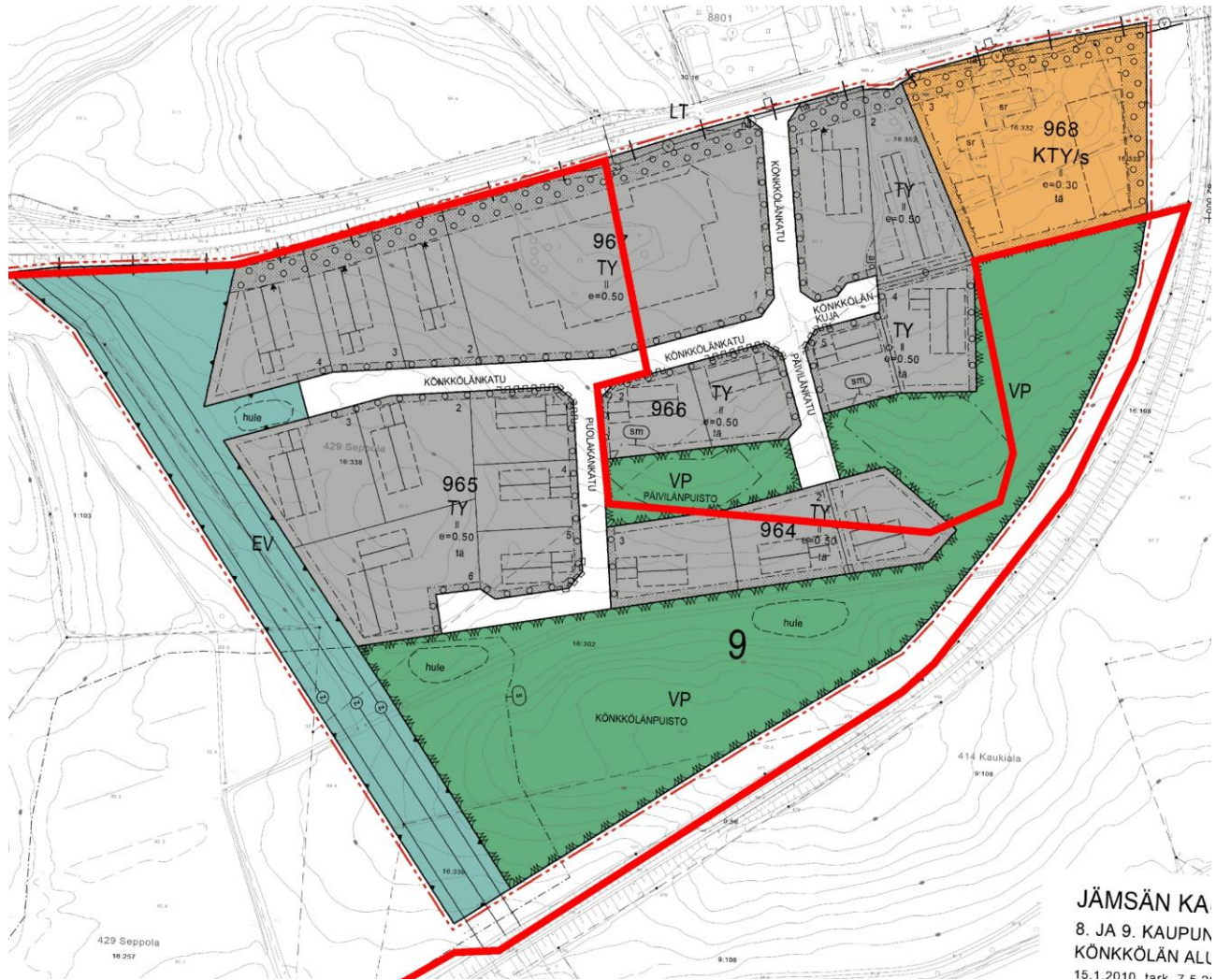
Kuva 13: Könkkölän asemakaava, hankealueen rajausta punaisella. Rajausta voi tarkentua prosessin aikana.
